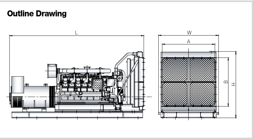
DATA Sheet 1500rpm, 50Hz
